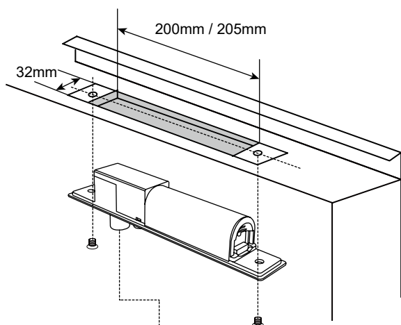
▲ Door Frame
